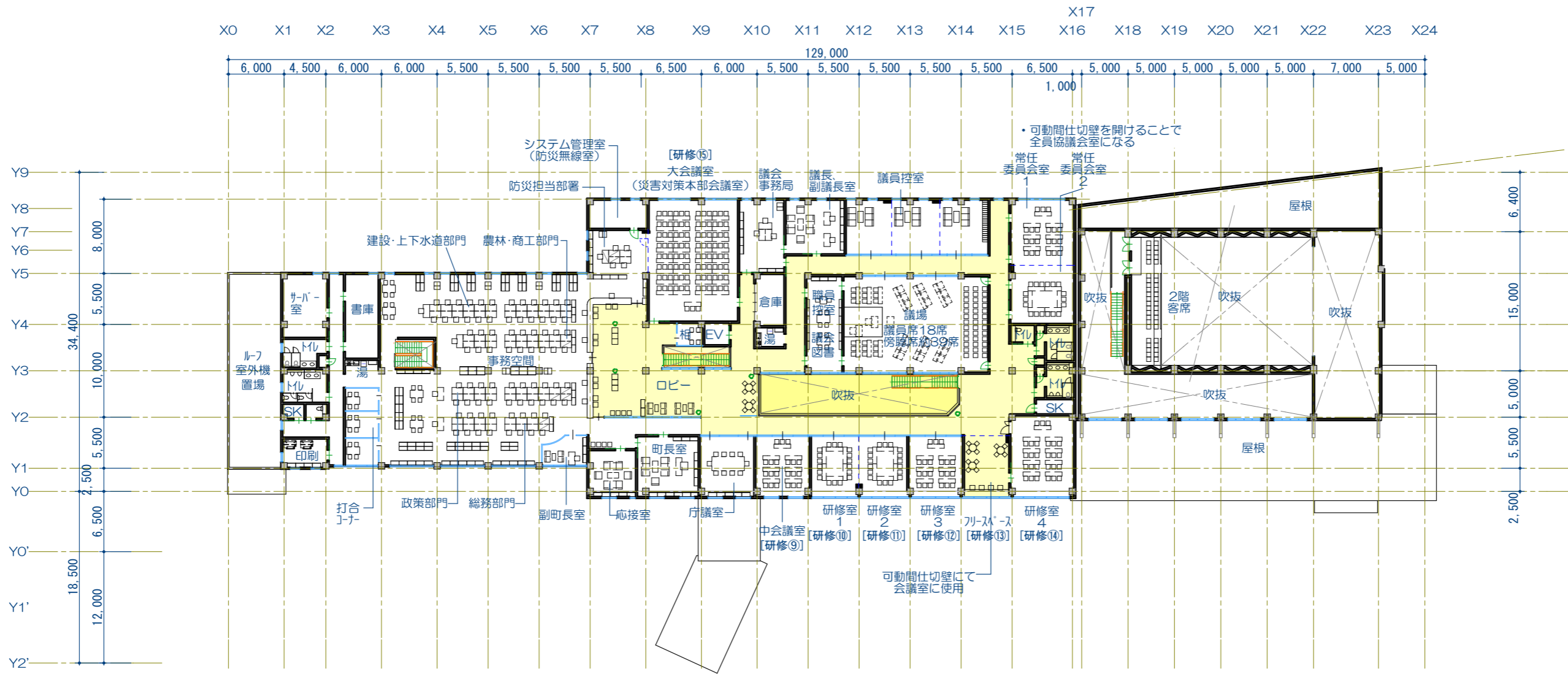
2階平面図 S=1:500
