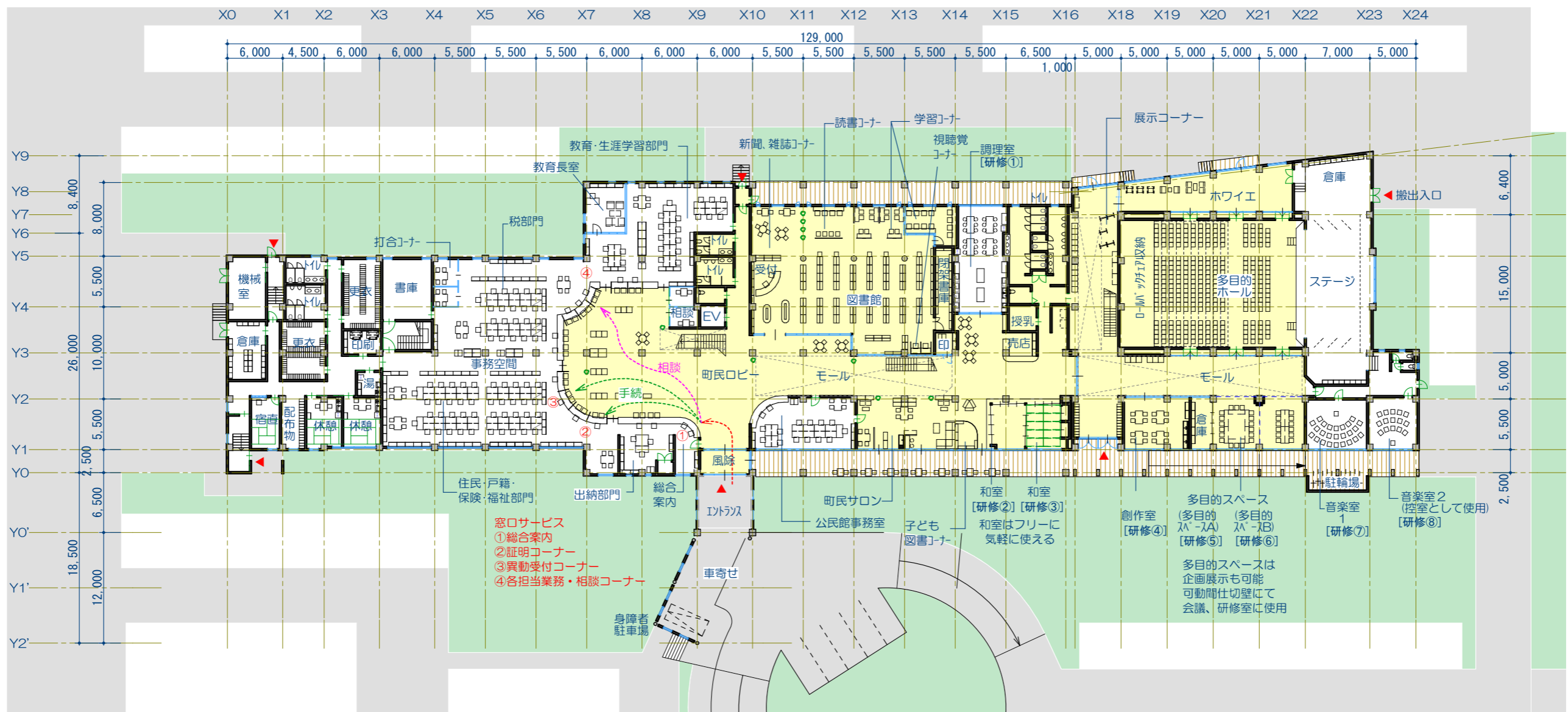
1階平面図 S=1:500
